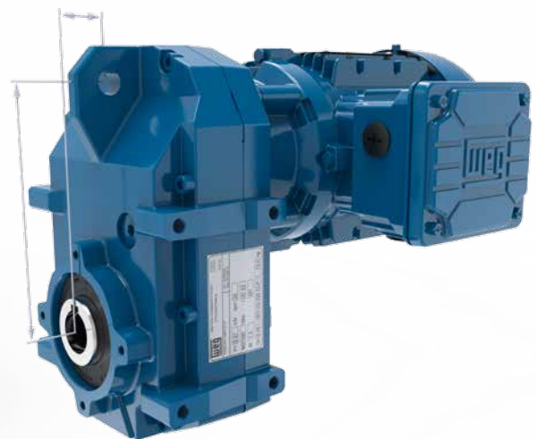
Schrumpfscheibe
