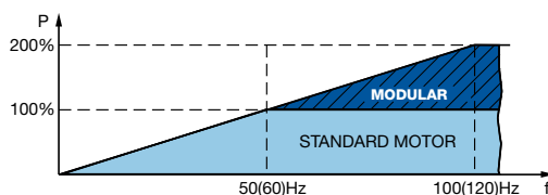
Doppelte Bemessungs-(Nenn-)leistung bei zweifacher Bemessungs-(Nenn-)drehzahl
