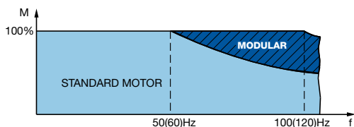
Bemessungs-(Nenn-)moment bis zur doppelten Bemessungs-(Nenn-)drehzahl
