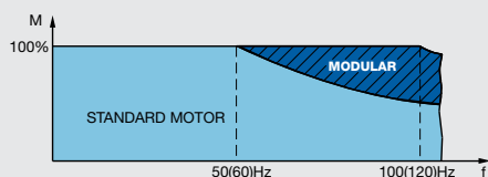
普通电机和模块化电机在双倍额定转速下的额定扭矩曲线
