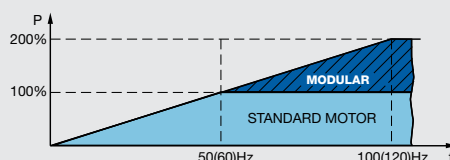
普通电机和模块化电机在双倍额定转速下的额定功率曲线
